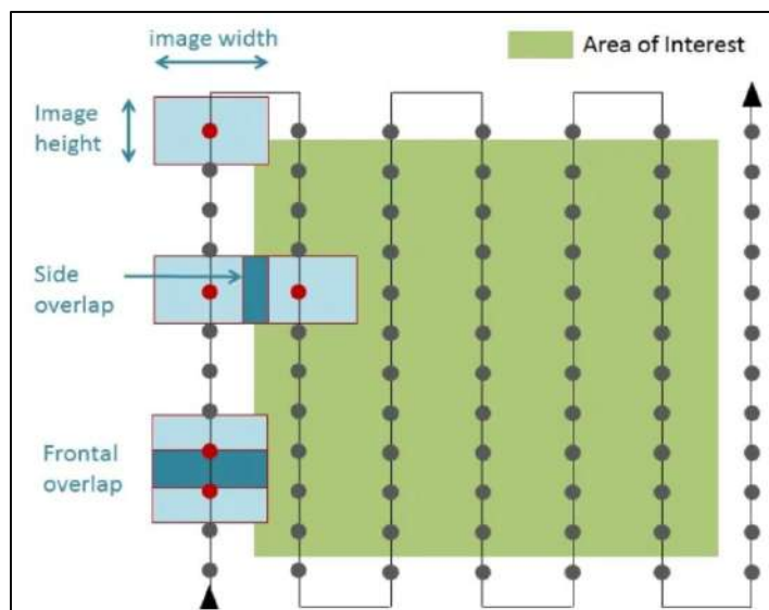
Figura 2: Modelo explicativo del solape lateral y frontal de las imágenes
